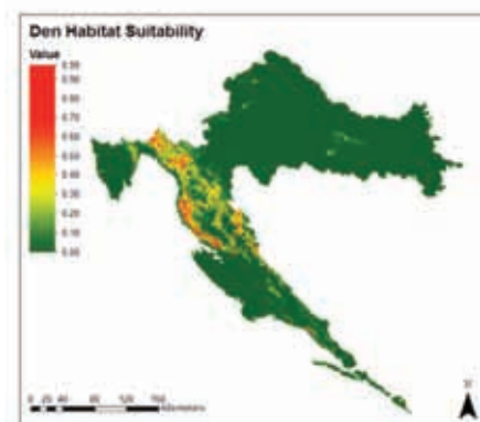
Slika 2. Karta vjerojatnosti pojavljivanja brloga medvjeda u Hrvatskoj na osnovi modeliranja 91 poznatog položaja brloga korištenjem 9 varijabli staništa.
