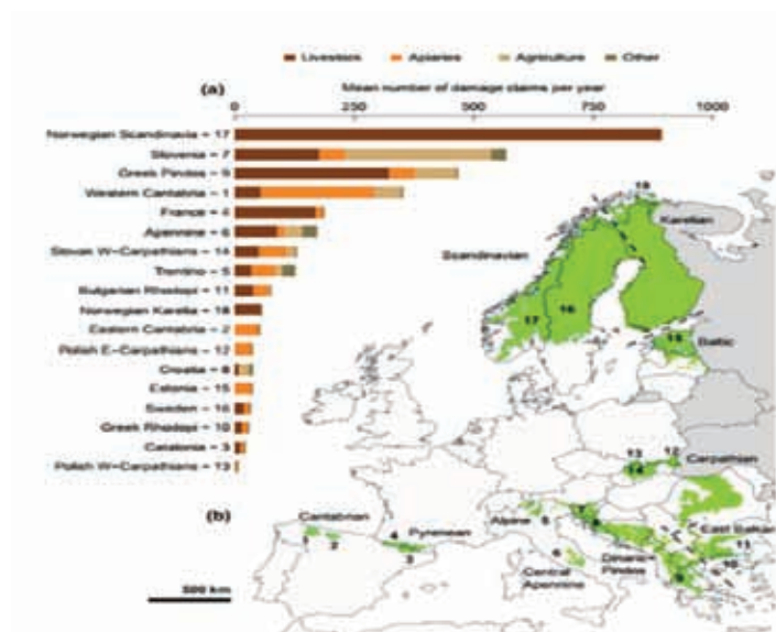
Slika 5. Prosječni broj oštetnih zahtjeva u 18 Europskih populacijskih segmenta u razdoblju 2005-2012.
